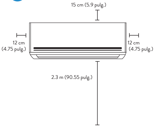
Seleccione el lugar de la instalación
